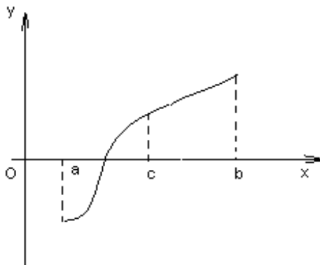
Рис 2.1. – функция f(x) меняет знак на отрезке [a;c]
