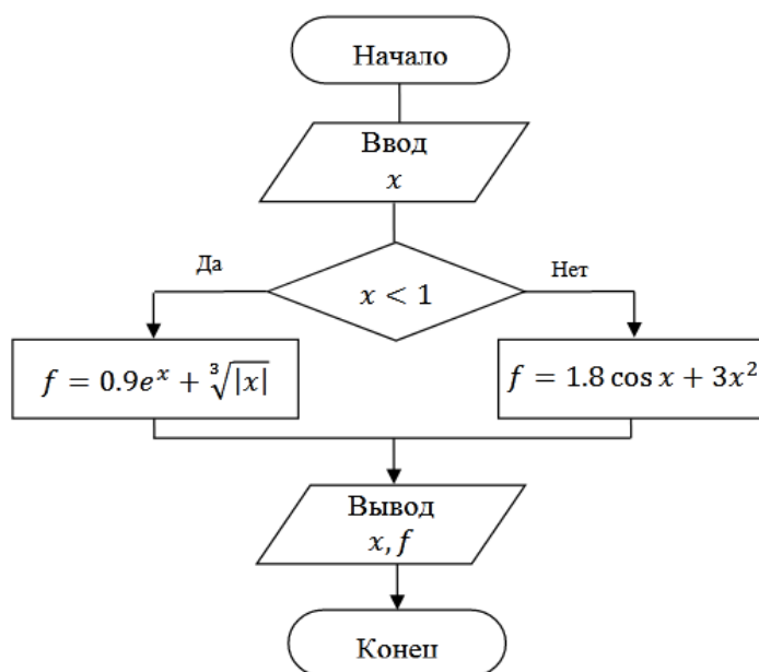
Блок-схема алгоритма
