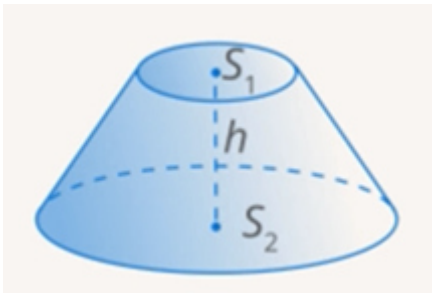
Рис. 18. Усеченная пирамида
