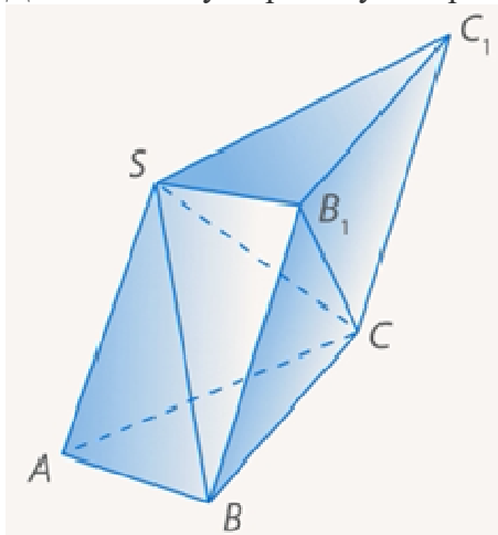
Рис. 6. Призма ABCSB_1C_1
