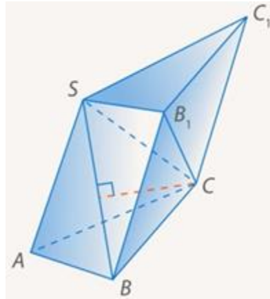
Рис. 8. Высота, проведенная к плоскости AB_1B
