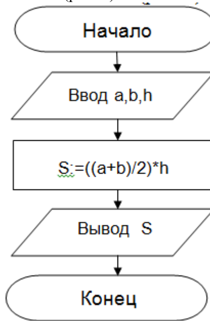
Рисунок 1. Блок-схема линейного алгоритма
