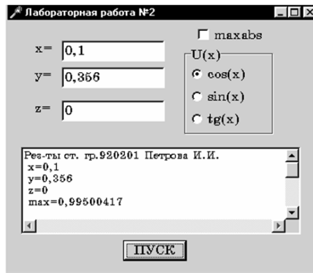
Рис. 5.1. Форма программы разветляющегося алгоритма
