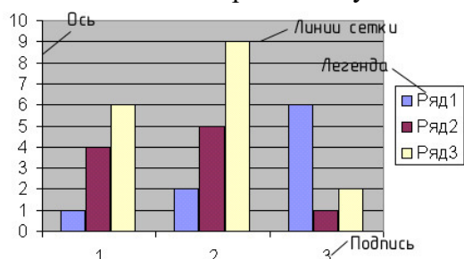
Рис. 2. Форматирование диаграммы
