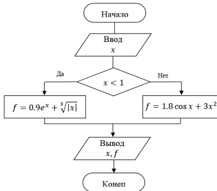
Блок-схема алгоритма
