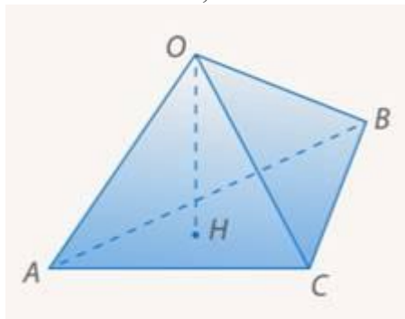
Рис. 1. Пирамида OABC
