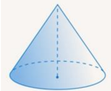
Рис. 15. Конус
