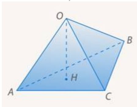
Рис. 1. Пирамида OABC
