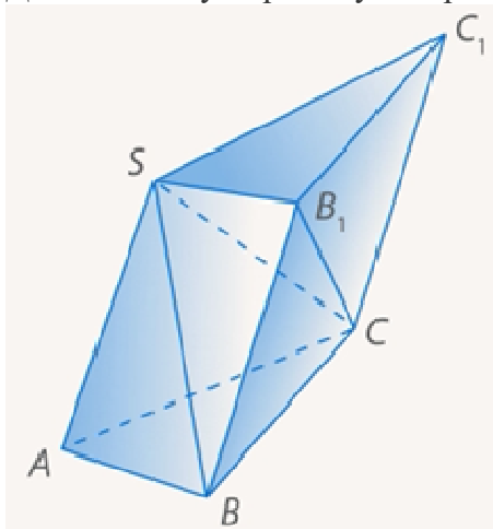
Рис. 6. Призма ABCB_1C_1
