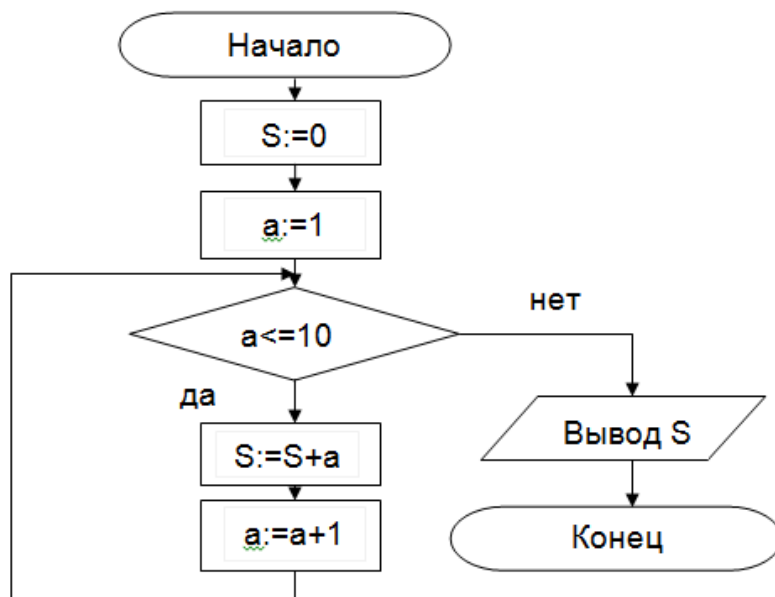
Рисунок 1. Циклический алгоритм с предусловием
