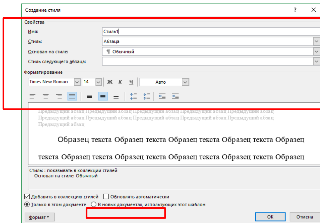
Рисунок 3 – Создание стиля
