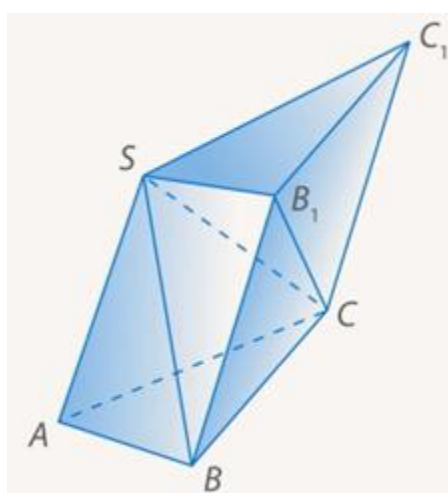
Рис. 6. Призма ABCSB_1C_1
